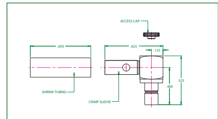
Right Angle Jack NM 3501 - 1630 - 5400
