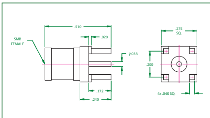
PC Mount Plug NM 3420 - 0031 - 5400
